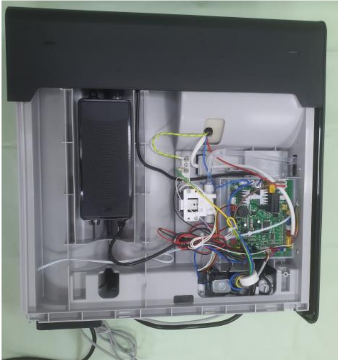
ERH-1005（内部结构）
